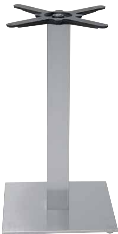
363 - 6032I (40 x 40 x H73 cm) kg 15 Base in acciaio inox satinato, piedini regolabili Stainless steel satin base
