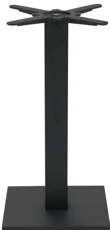
365 - 340N (40 x 40 x H72 cm) kg 15 Base in acciaio verniciato, piedini regolabili Steel base, powder coating
