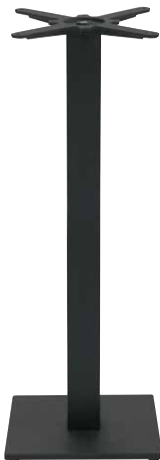
749 - 33940H (40 x 40 x H108 cm) kg 17 Base in acciaio verniciato, piedini regolabili Steel base, powder coating
