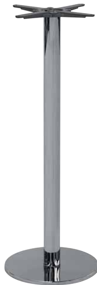
399 - 6029C (Ø 40 x H110 cm) kg 13,5 Base in acciaio cromato, piedini regolabili Chromated steel base
